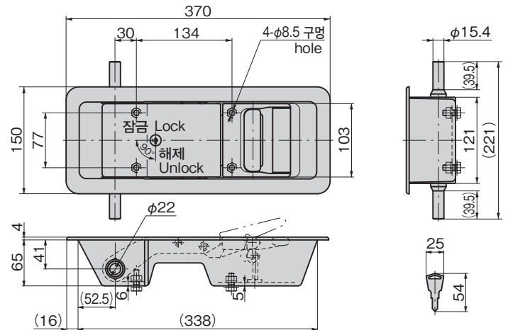
[FA-877-3-JL] 안전 누름 버튼 부착 이중 록 타입 The double locked-type with safety push button.
