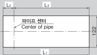
패널 구멍 치수 Panel drilling dimensions
