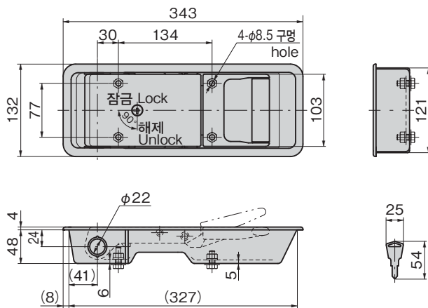
[FA-877-1] 리어 도어 타입 Rear door type
