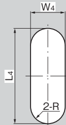
패널 구멍 치수 Panel drilling dimensions
