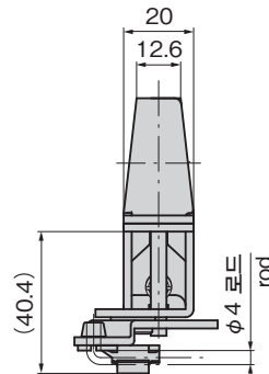
사용 로드 접속부 가공도 Figure of machining rod for connection
