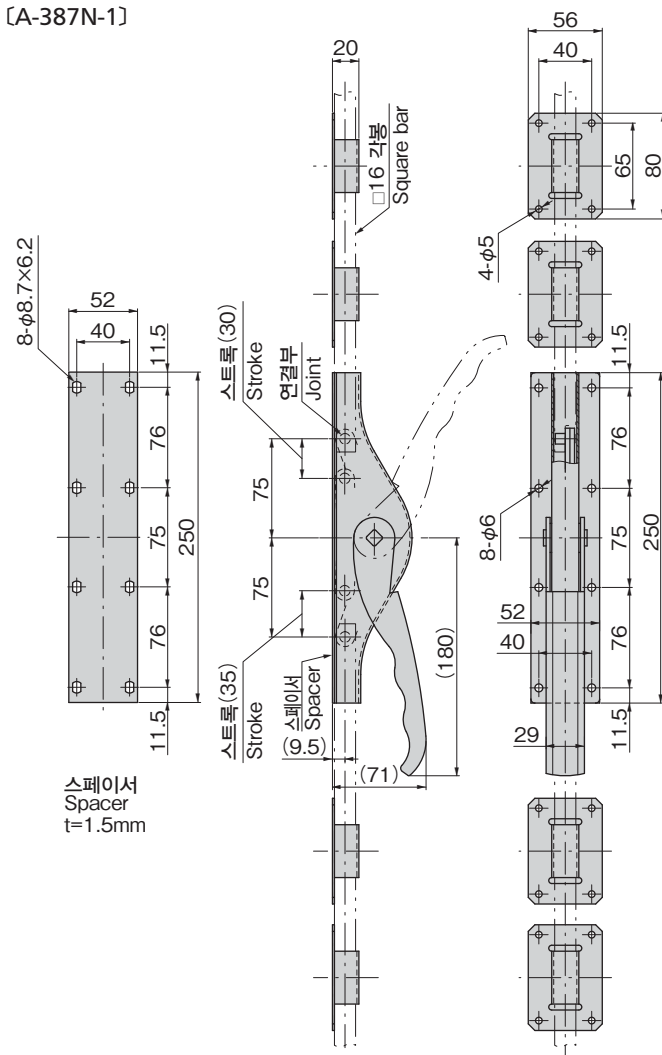
각봉 가공 치수 참고 예 Rod shortening dimensions (Reference)
