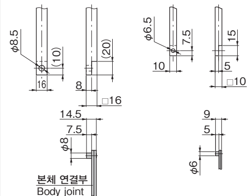
각봉 가공 치수 참고 예 Rod shortening dimensions (Reference)
