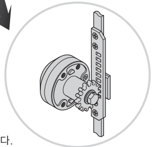
■핸들부 Handle
