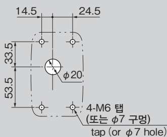
패널 구멍 치수 Panel drilling dimensions
