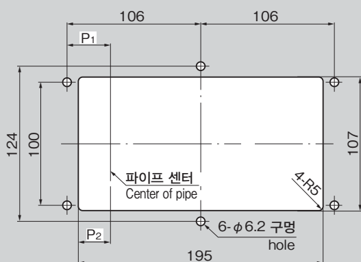
패널 구멍 치수 Panel drilling dimensions (FA-816-1, FA816-2)
