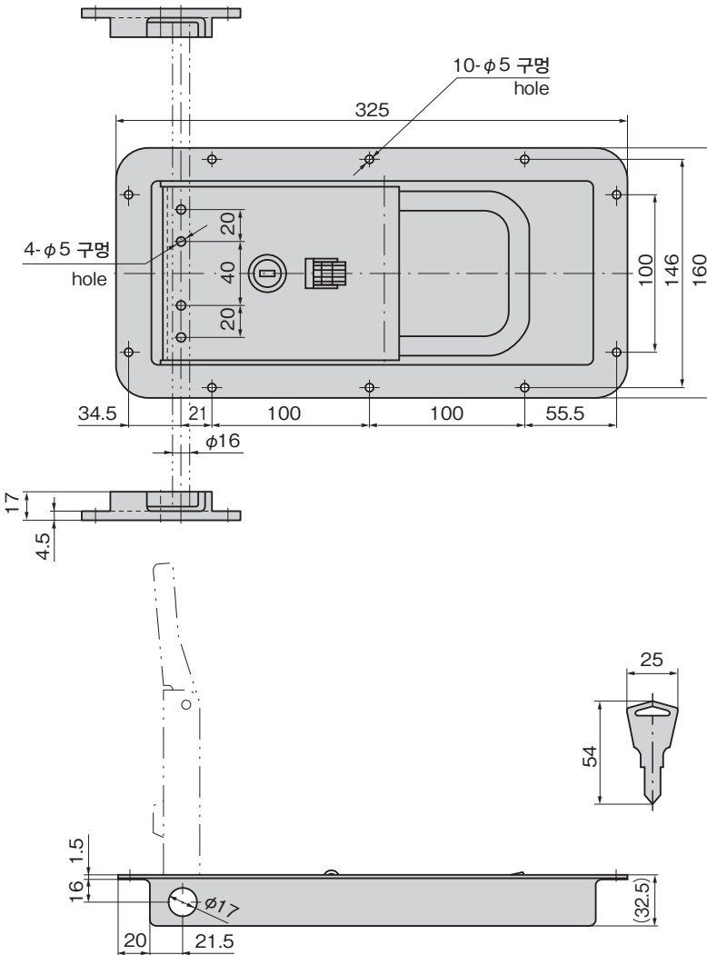
키 No.T0230 Key
