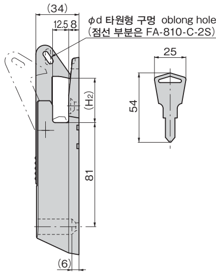
적용 핸들 단면 치수(최대) Applicable handle cross section dimension (max.)
