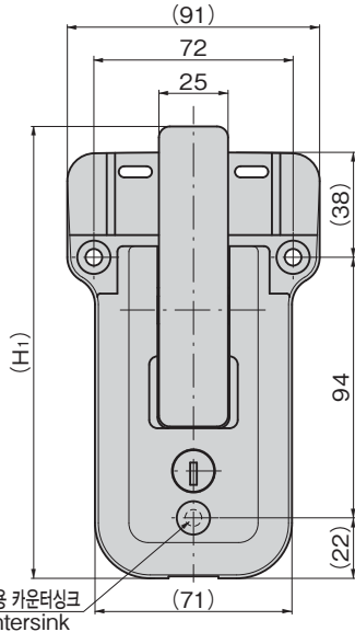
적용 핸들 단면 치수(최대) Applicable handle cross section dimension (max.)
