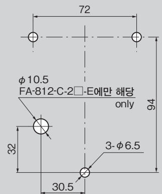
패널 구멍 치수 Panel drilling dimensions
