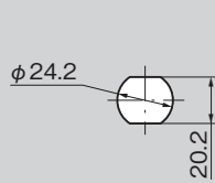
패널 구멍 치수 Panel drilling dimensions
