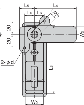
패널 구멍 치수 Panel drilling dimensions
