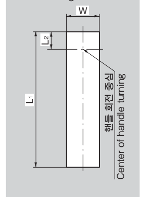
패널 구멍 치수 Panel drilling dimensions
