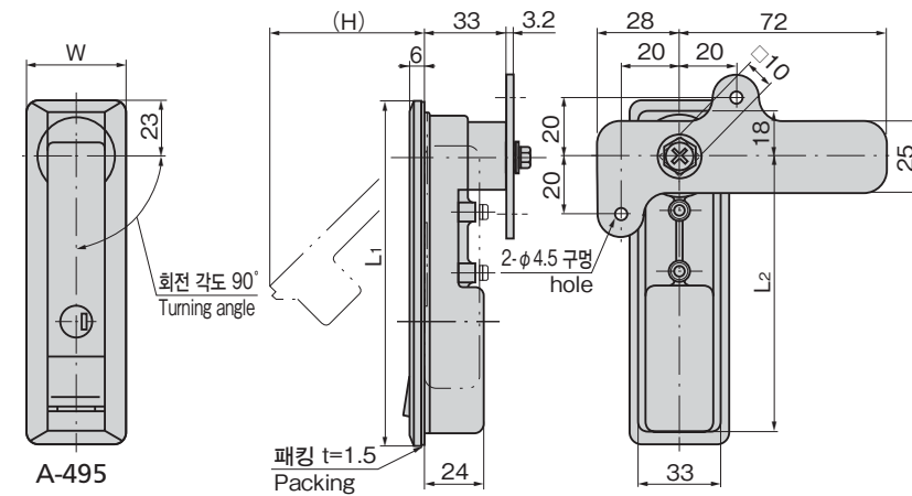
A-495-2-TAK60
