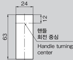
패널 구멍 치수 Panel drilling dimensions
