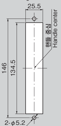
패널 구멍 치수 Panel drilling dimensions
