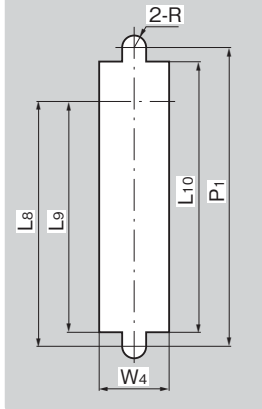
패널 구멍 치수 Panel drilling dimensions
