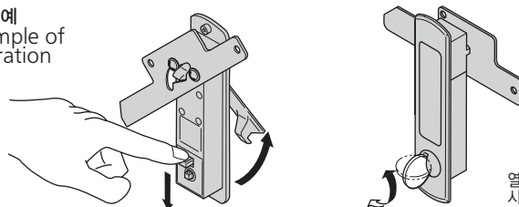
내부 해제 레버 Inside emergency lock-release lever
