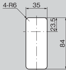
패널 구멍 치수 Panel drilling dimensions
