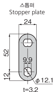
패널 구멍 치수 Panel drilling dimensions
