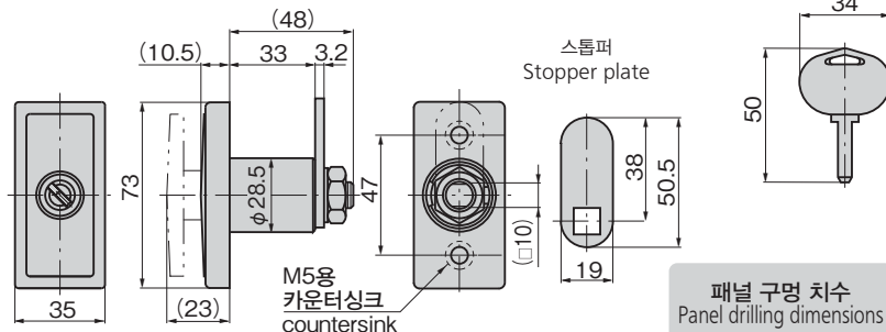
키 No. Z00288 Key
