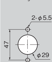
패널 구멍 치수 Panel drilling dimensions
