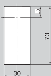
패널 구멍 치수 Panel drilling dimensions
