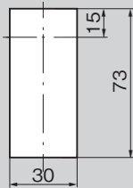
패널 구멍 치수 Panel drilling dimensions
