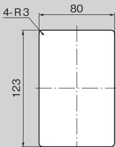
패널 구멍 치수 Panel drilling dimensions
