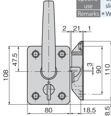
적용 도어 판 두께 22~26 Applicable door thickness
