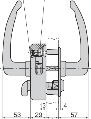
적용 도어 판 두께 22~26 Applicable door thickness
