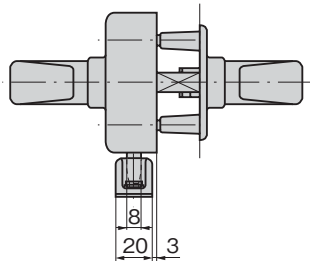
M5나사 (부속되어 있지 않습니다) screw (Not included)
