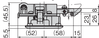
조정 마진 58 (-7~+9) Adjustment margin
