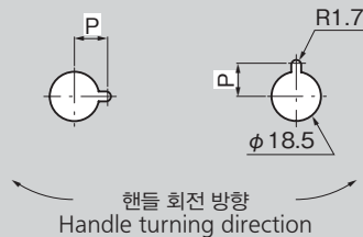
패널 구멍 치수 Panel drilling dimensions
