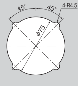
패널 구멍 치수 Panel drilling dimensions
