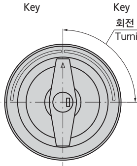
키 No.TAK60 Key
