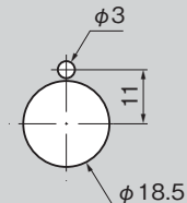
패널 구멍 치수 Panel drilling dimensions
