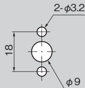
패널 구멍 치수 Panel drilling dimensions
