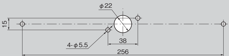
패널 구멍 치수 Panel drilling dimensions
