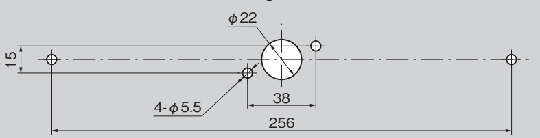
패널 구멍 치수 Panel drilling dimensions
