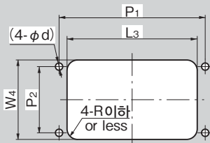
패널 구멍 치수 Panel drilling dimensions
