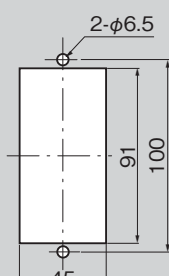
패널 구멍 치수 Panel drilling dimensions
