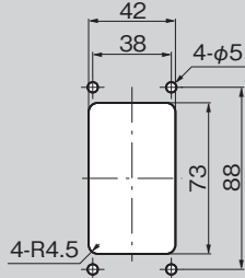
패널 구멍 치수 Panel drilling dimensions
