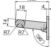
단면도 A-A Cross-section A-A (62)
