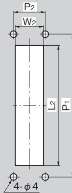
패널 구멍 치수 Panel drilling dimensions
