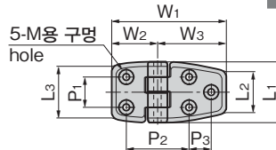
BP-19-2-2-S 접시머리 나사용 For countersink screw
