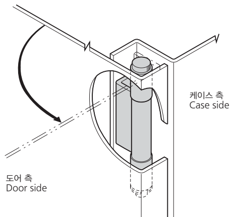
사용 예 Example of application
