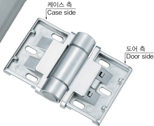
커버 미장착 시 When cover unmounted
