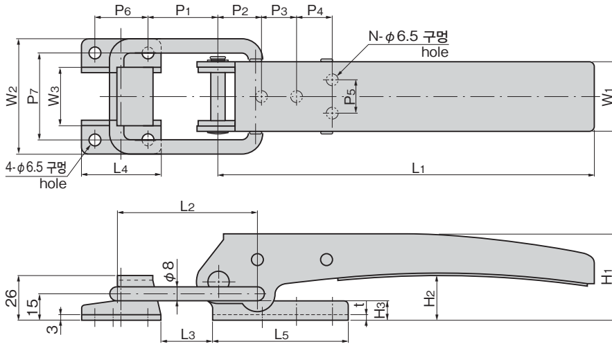
※본 그림은 조임 마진 0mm인 경우입니다.※Drawings show the tightening margin of 0mm.
