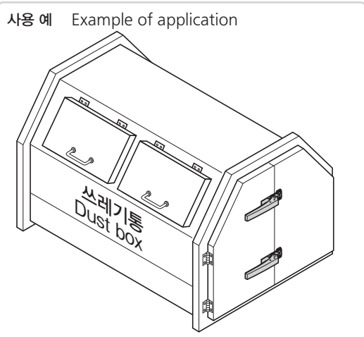
※본 그림은 조임 마진 0mm인 경우입니다.※Drawings show the tightening margin of 0mm.
