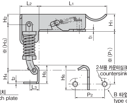
잠금 해제 레버 Lock release lever
