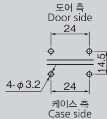
패널 구멍 치수 Panel drilling dimensions
