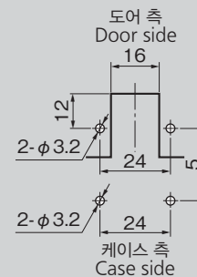
패널 구멍 치수 Panel drilling dimensions
