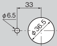
패널 구멍 치수 Panel drilling dimensions
