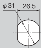
패널 구멍 치수 Panel drilling dimensions
