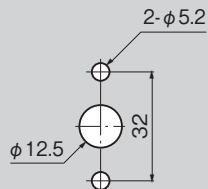
패널 구멍 치수 Panel drilling dimensions
