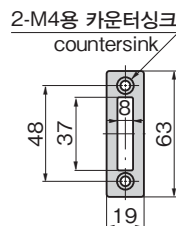
캐치 Striker
