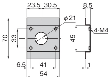
부착 쇠장식 Installing plate
