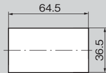
패널 구멍 치수 Panel drilling dimensions
